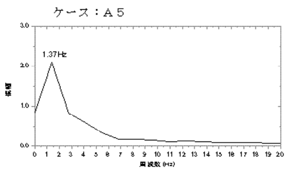
図-2.5.8(b) 軸重変動波形の周波数特性 (段差高さ 100mm 速度 10km/h 1 回目走行)
