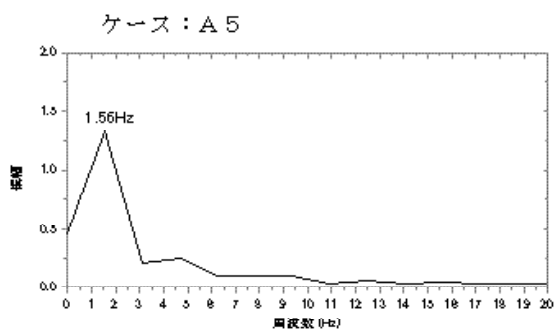
図-2.5.7(b) 軸重変動波形の周波数特性 (段差高さ 80mm 速度 10km/h 1回目走行)
