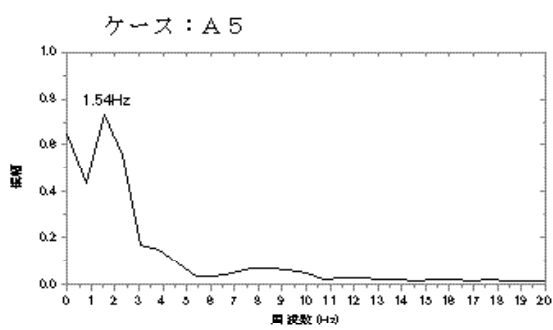
図-2.5.4(b) 軸重変動波形の周波数特性 (段差高さ 80mm 速度 5km/h 1 回目走行)
