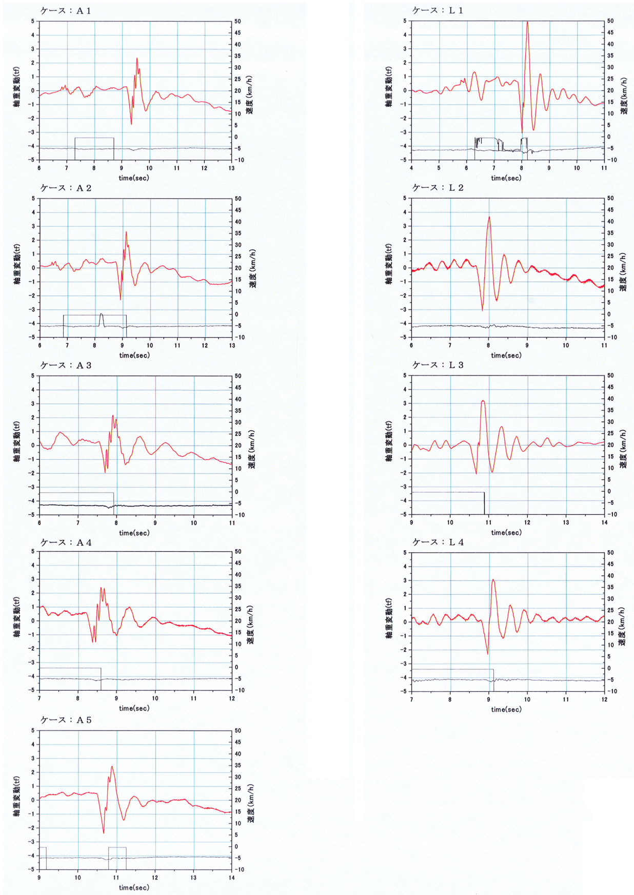
図-2.5.3(a) 人工段差落下試験軸重波形 (段差高さ 60mm 速度 5km/h 1 回目走行)
