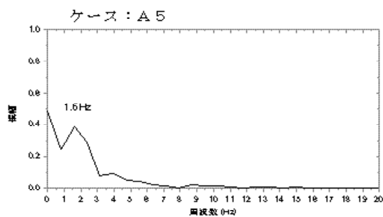
図-2.5.3(b) 軸重変動波形の周波数特性 (段差高さ 60mm 速度 5km/h 1 回目走行)
