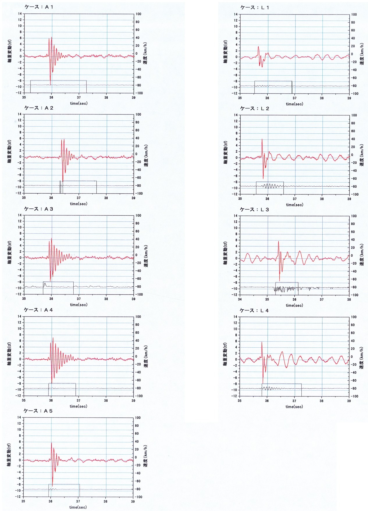
図-2.4.18 (b) 単独段差試験軸重波形 (段差高さ 20mm [斜路あり] 速度 80km/h 1 回目走行)
