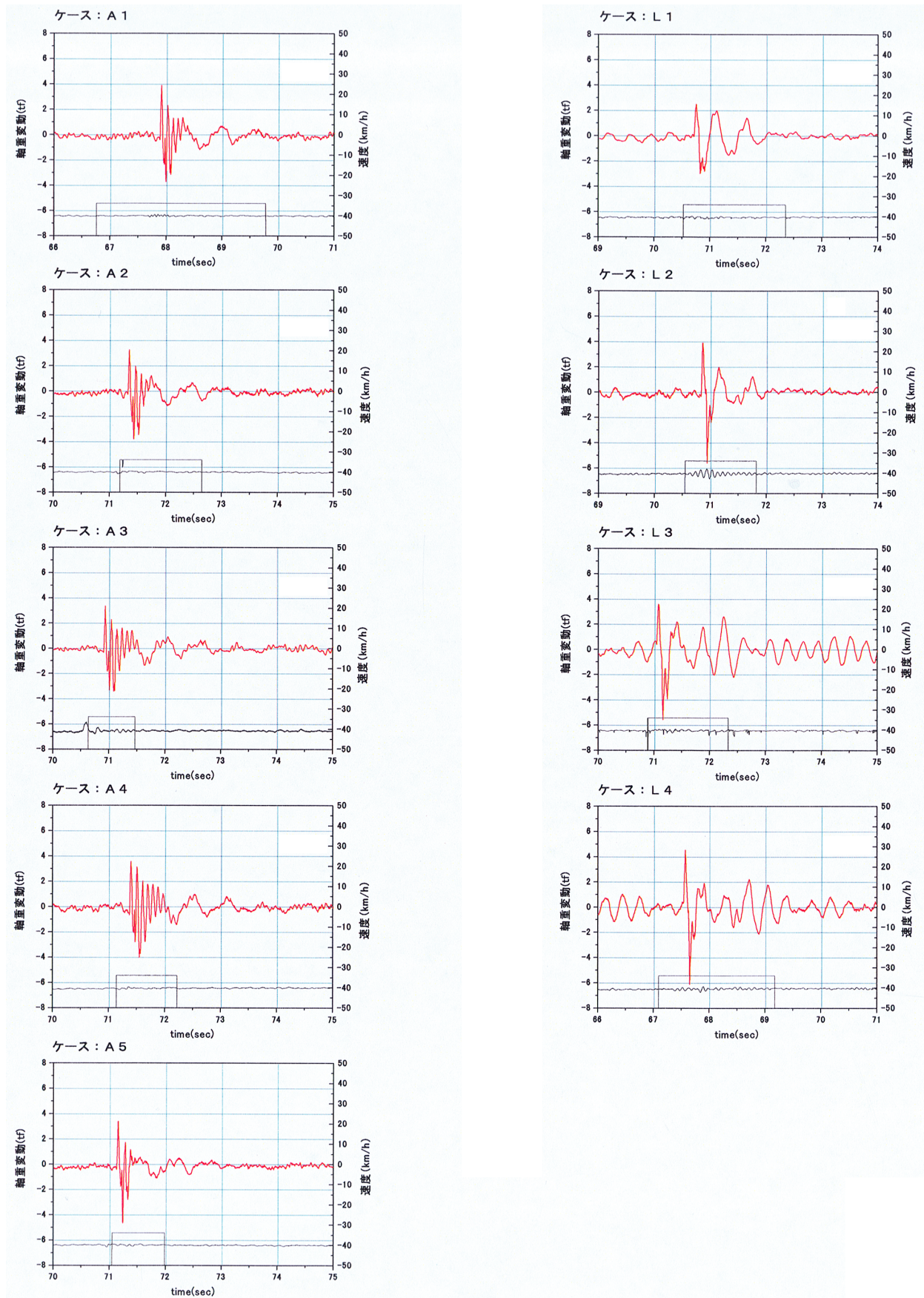
図-2.4.18(a) 単独段差試験軸重波形 (段差高さ 20mm [斜路あり] 速度 40km/h 1 回目走行)
