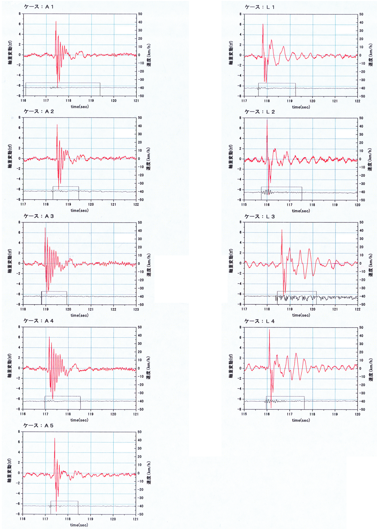
図-2.4.16(a) 単独段差試験軸重波形 (段差高さ 30mm [斜路なし] 速度 40km/h 1 回目走行)
