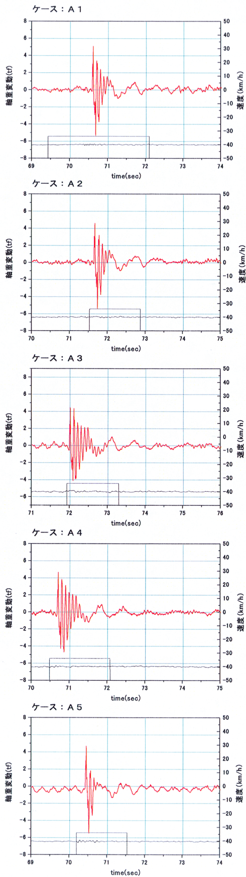
図-2.4.15 (a) 単独段差試験軸重波形 (段差高さ 20mm [斜路なし] 速度 40km/h 1 回目走行)
