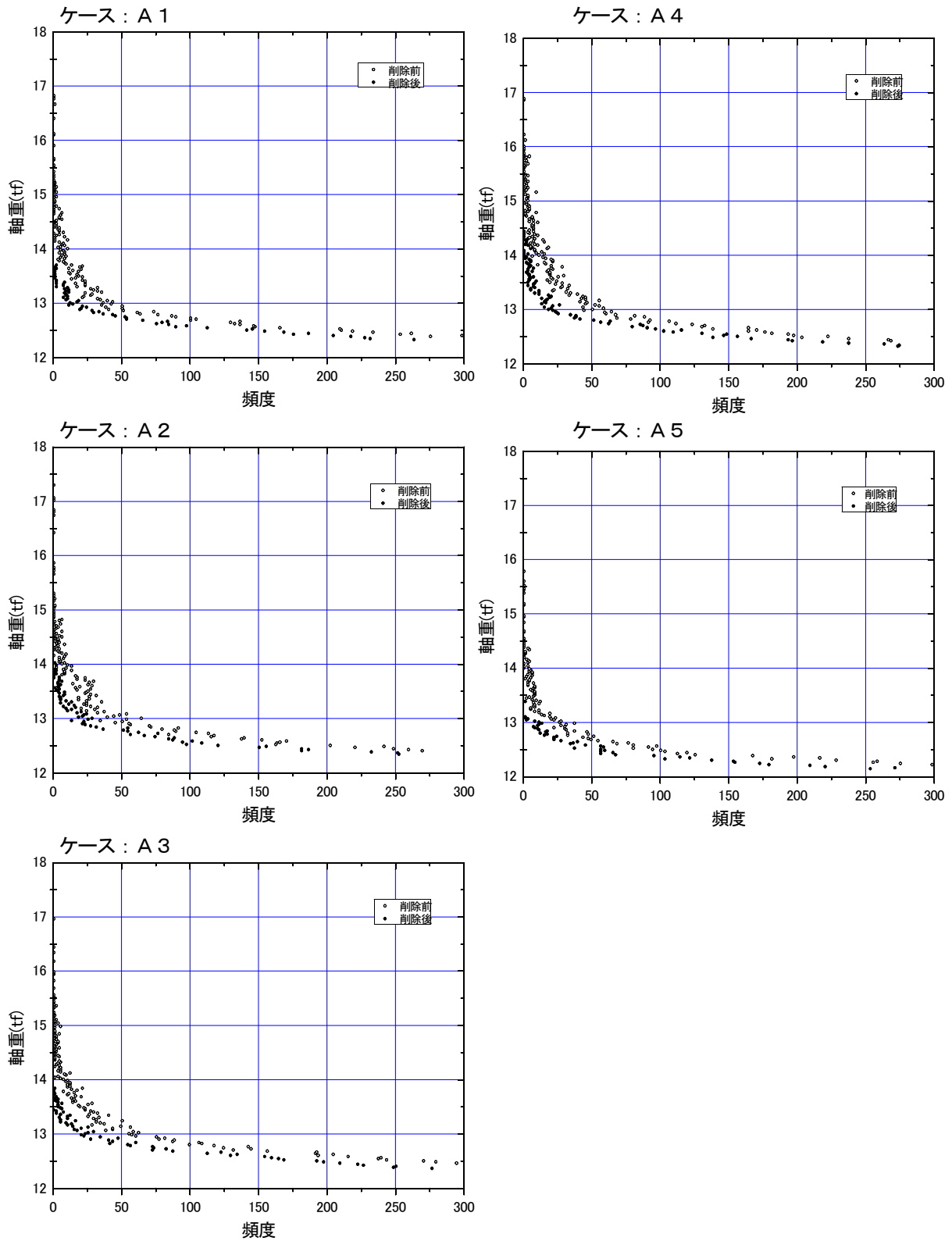
図-2.3.31(a) 一般道走行試験軸重頻度分布 (エアサス、特異区間データ削除前後比較 (拡大)、全3回分データ)
