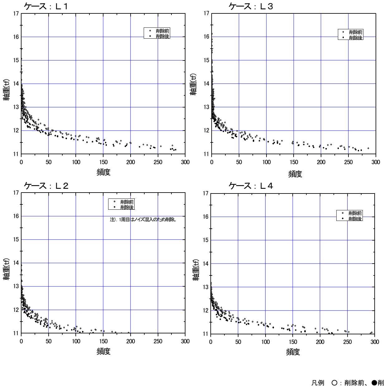
図-2.3.31 (b) 一般道走行試験軸重頻度分布 (リーフサス、特異区間データ削除前後比較 (拡大)、全3回分データ)
