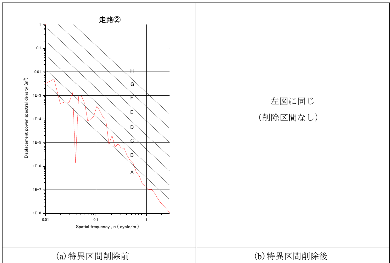
図-2.3.13 路面の周波数特性 (P S D、基本計測区間②)
