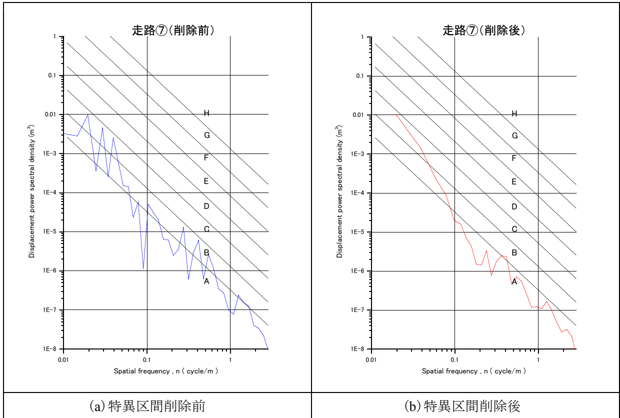
図-2.3.18 路面の周波数特性 (P S D、基本計測区間⑦)
