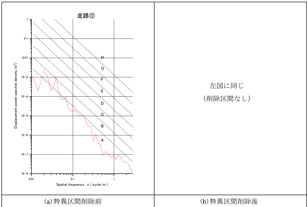
図-2.3.23 路面の周波数特性 (PSD、基本計測区間⑫)
