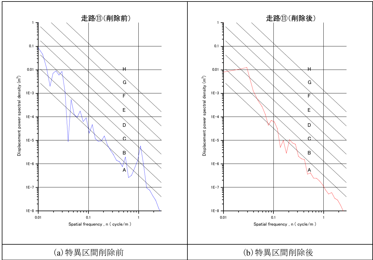
図-2.3.22 路面の周波数特性 (PSD、基本計測区間⑪)
