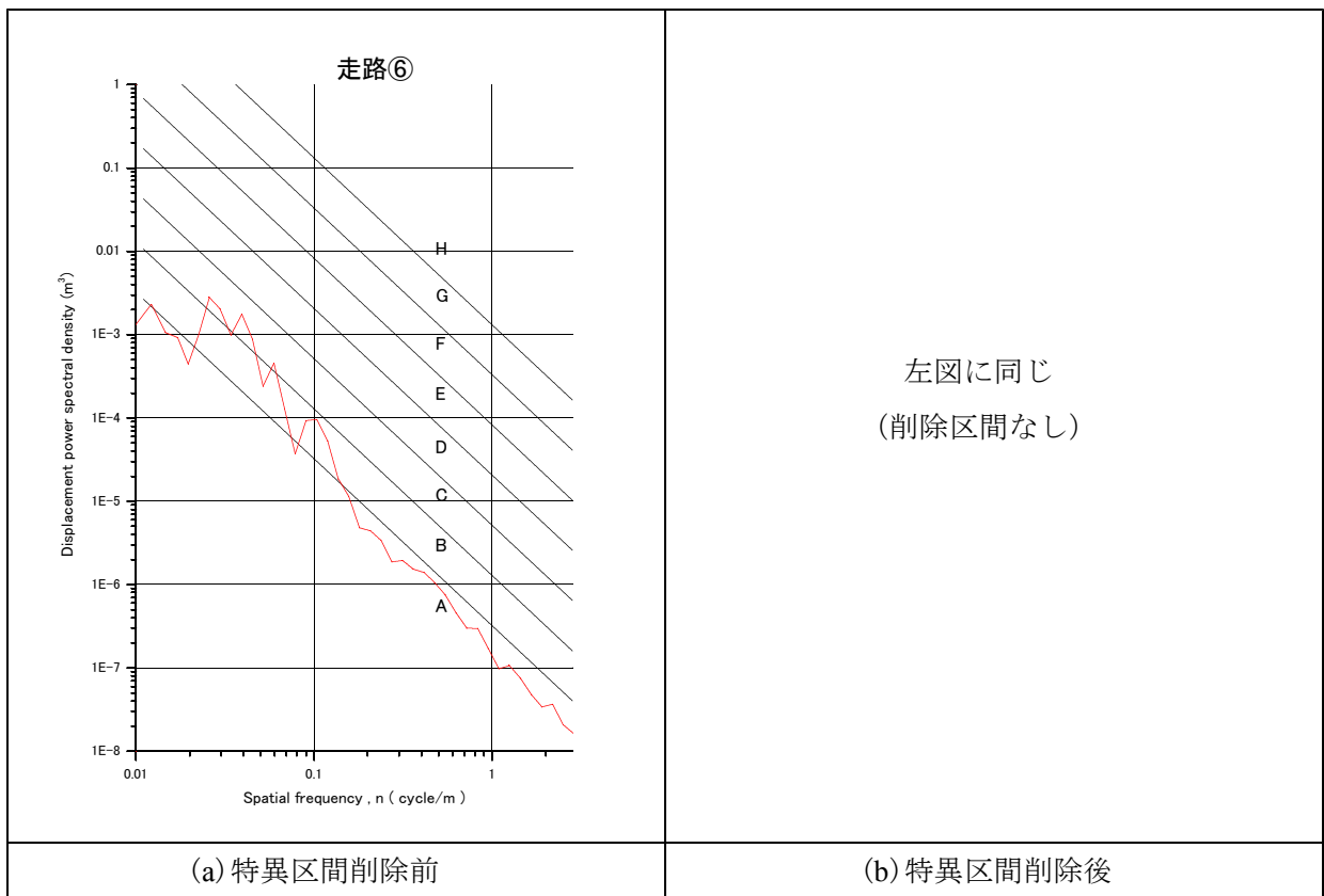
図-2.3.17 路面の周波数特性 (PSD、基本計測区間⑥)
