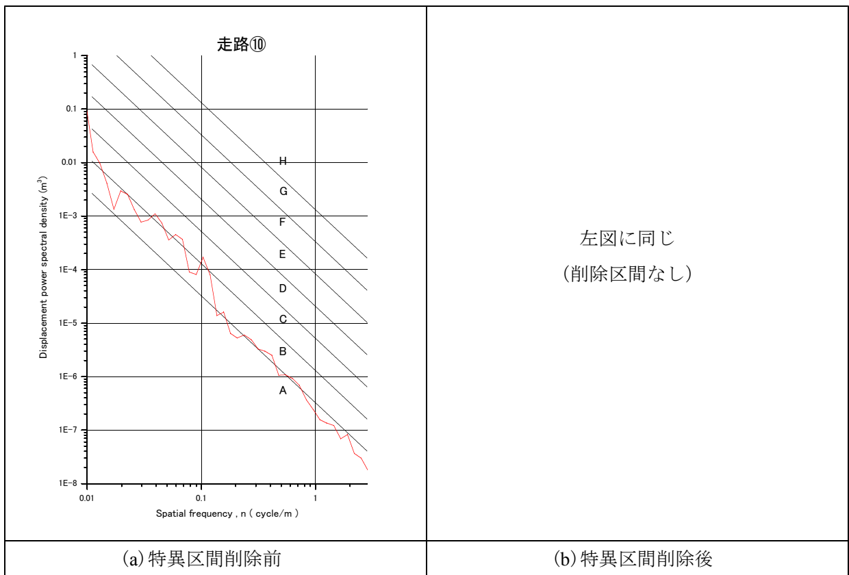
図-2.3.21 路面の周波数特性 (P S D、基本計測区間⑩)
