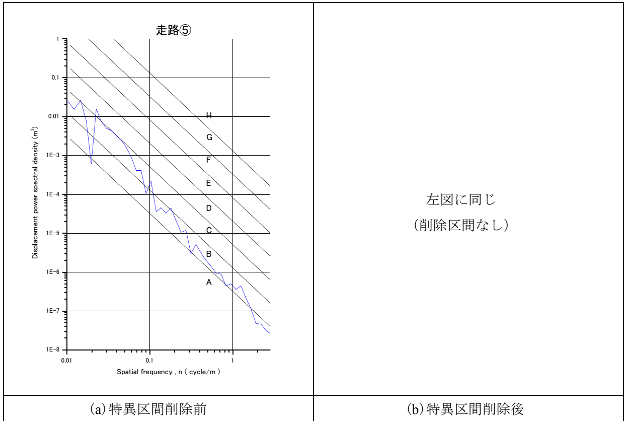
図-2.3.16 路面の周波数特性 (PSD、基本計測区間⑤)
