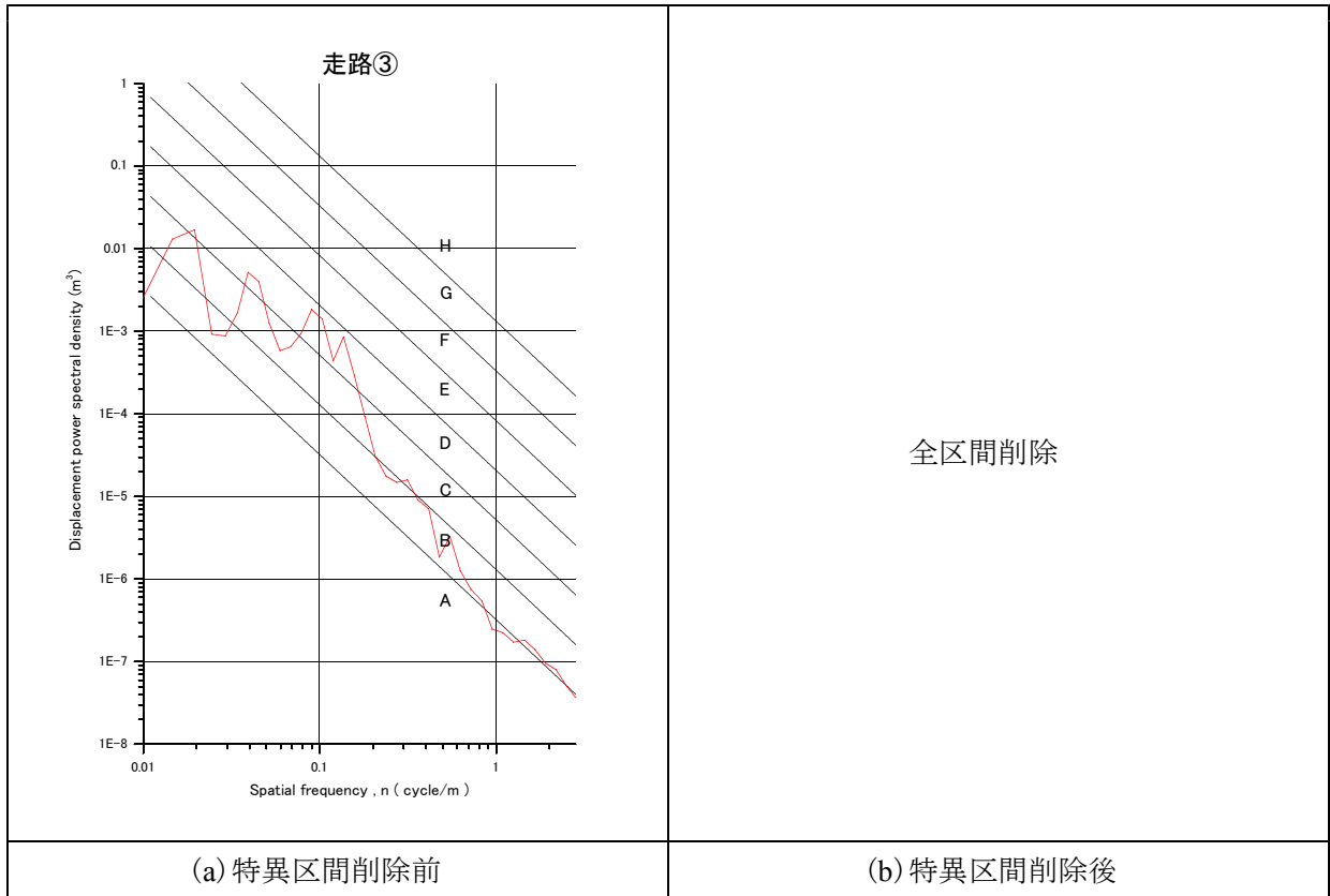
図-2.3.14 路面の周波数特性 (P S D、基本計測区間③)
