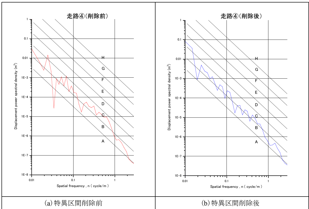
図-2.3.15 路面の周波数特性 (P S D、基本計測区間④)
