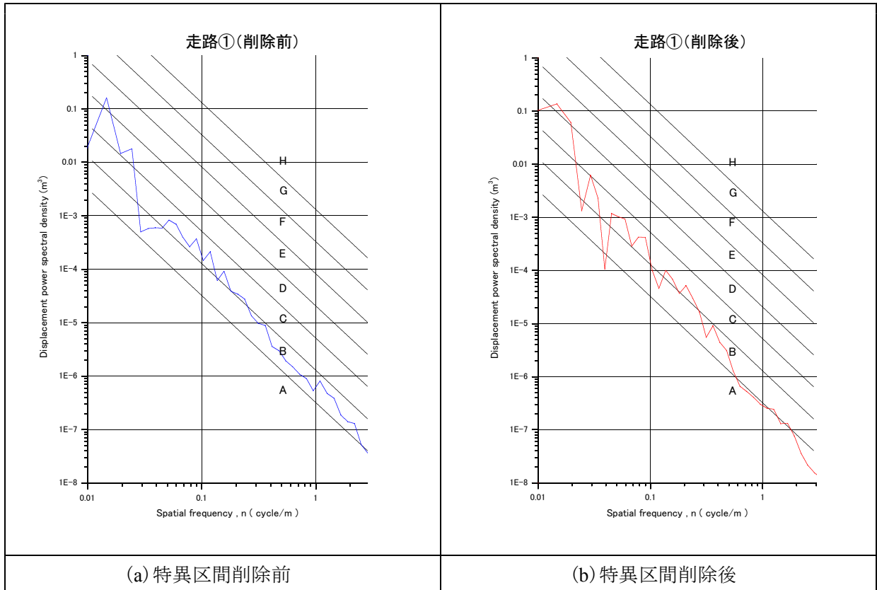
図-2.3.12 路面の周波数特性 (P S D、基本計測区間①)
