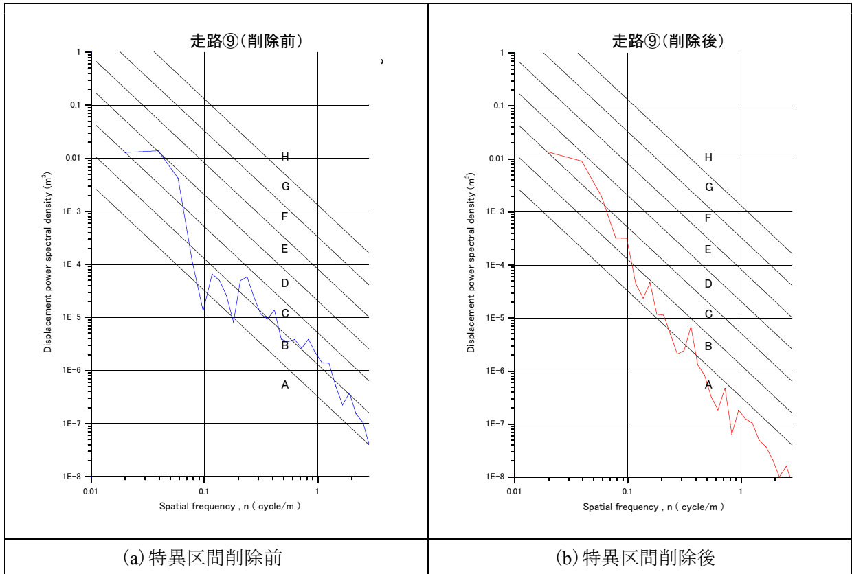
図-2.3.20 路面の周波数特性 (P S D、基本計測区間⑨)
