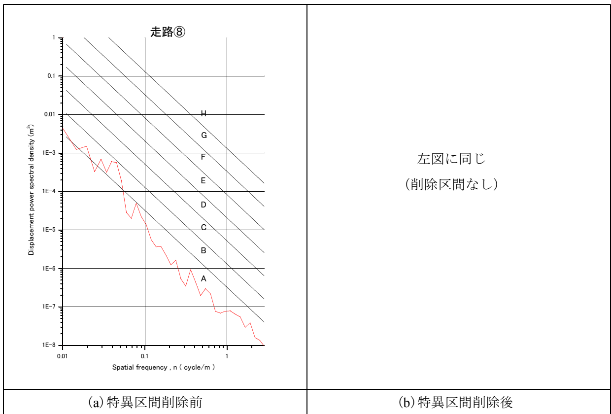
図-2.3.19 路面の周波数特性 (P S D、基本計測区間⑧)
