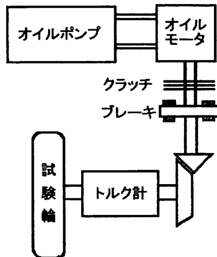
図-1.4 トルク計による検出装置
