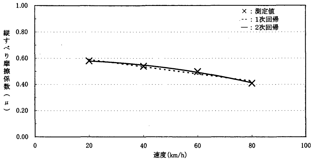
図—4. 5 速度とすべり摩擦係数の関係 [縦すべり摩擦係数(BF)] [近畿技術事務所測定車、コンクリート研磨路面(標準路)、リブタイヤ]
