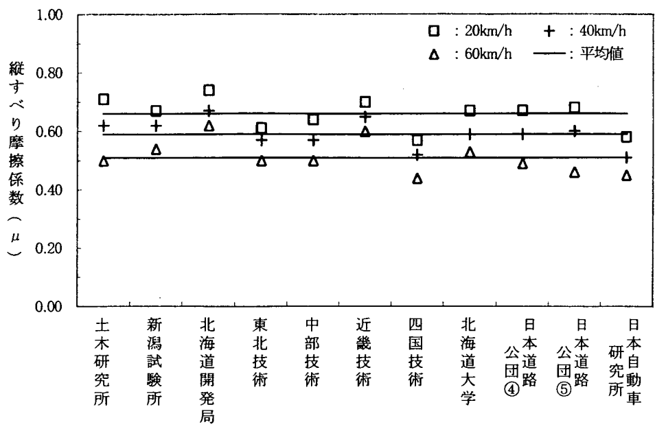
図-3.7.1 測定車別縦すべり摩擦係数 (BF) [アスファルト路面 (高μ路)・リブタイヤ]
