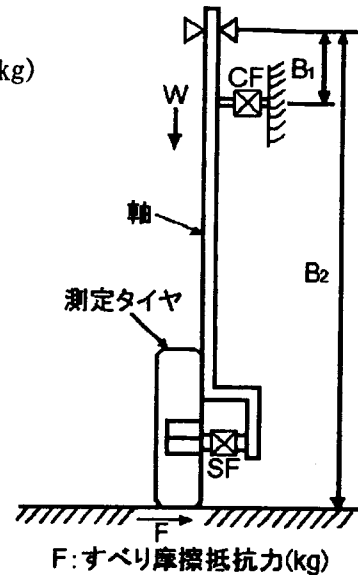
図-2. 6 垂直昇降式すべり計(横すべり)
