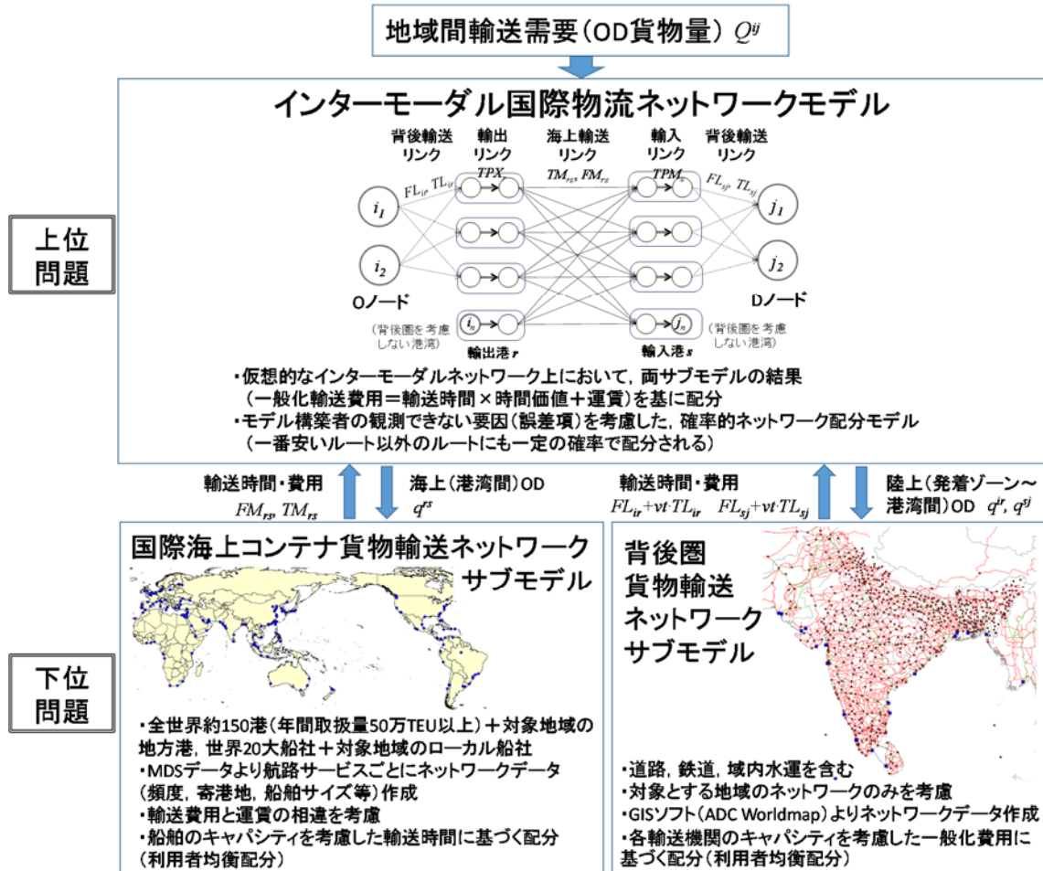
図-2 モデルの全体構成
