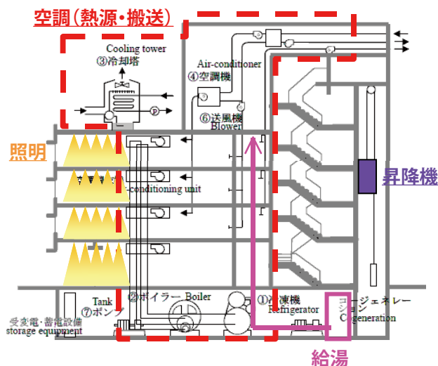
図 建築の評価対象設備システム(例)
