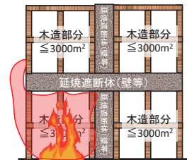
図-2 壁等の延焼遮断性能評価の改良
