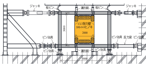
図-1 CLT壁+S架構試験体の水平加力実験
