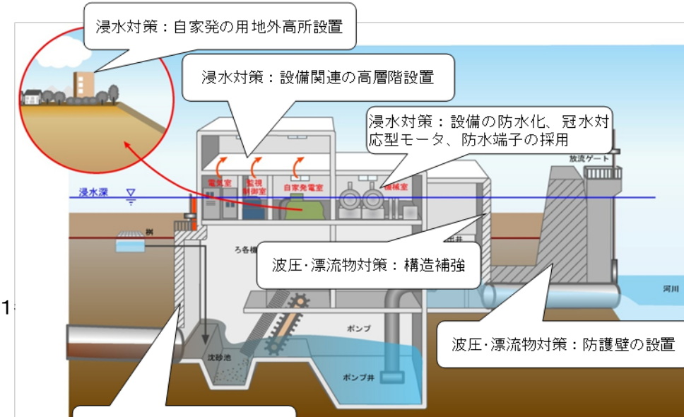
波圧・漂流物対策：構造補強
