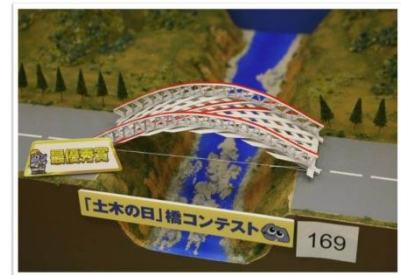
メッシュなブリッジ
