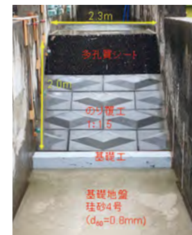
●法尻の補強に関する水理実験
