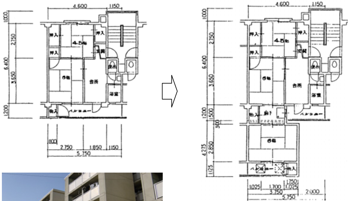
従前バルコニーの一部を廊下にし、6畳1室を南に増築(公営住宅の例)
