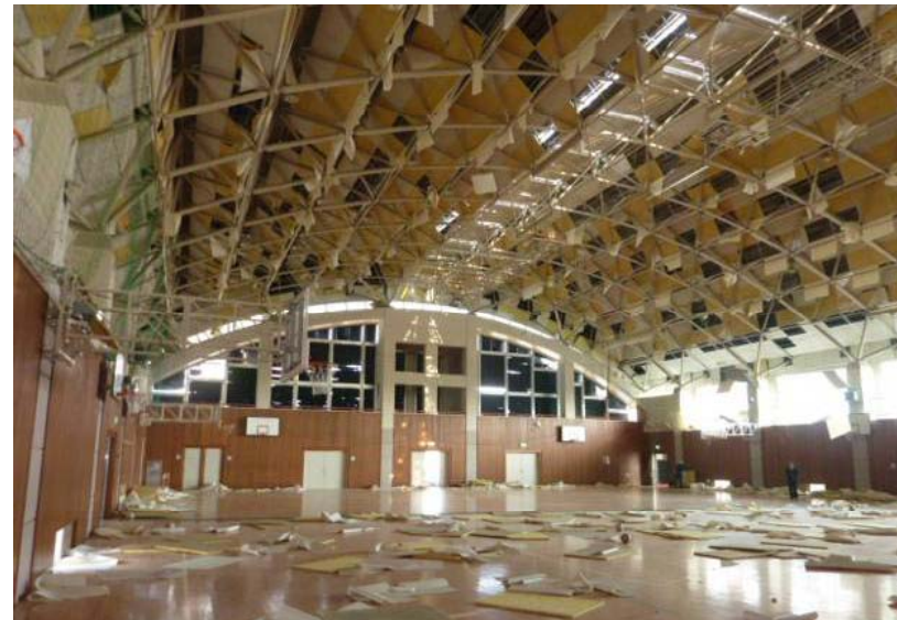
システム天井のグラスウール板の脱落
